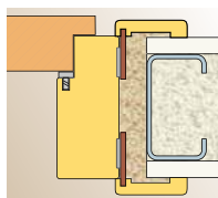
Монтаж с пена на гипсо-картонена стена
