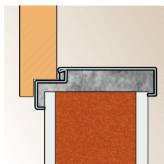
Каса ъглова голяма – На стена с дебелина 100 мм
