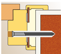
Монтаж с пяна и котви на тухлена стена
