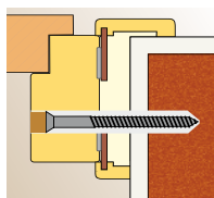
Монтаж с пена и котва на тухлена стена
