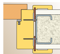
Монтаж с винтове на гипсо-картонена стена
