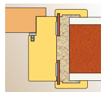
Монтаж с пена на тухлена стена
