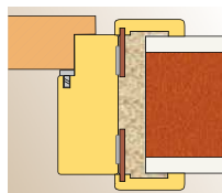
Монтаж с пяна на тухлена стена
