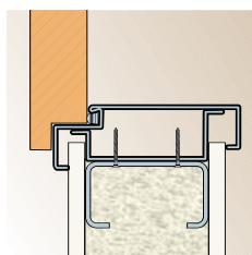
Каса ъглова голяма на гипсо-картонена стена
