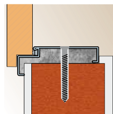
Каса ъглова голяма на стена с дебелина по-голяма от 100 мм
