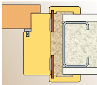
Монтаж с пяна на стена гипсо-картонена
